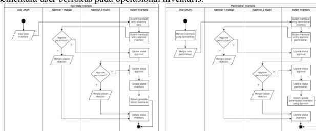
Gambar 3.4 Activity Diagram Input dan Pemindahan Inventaris
